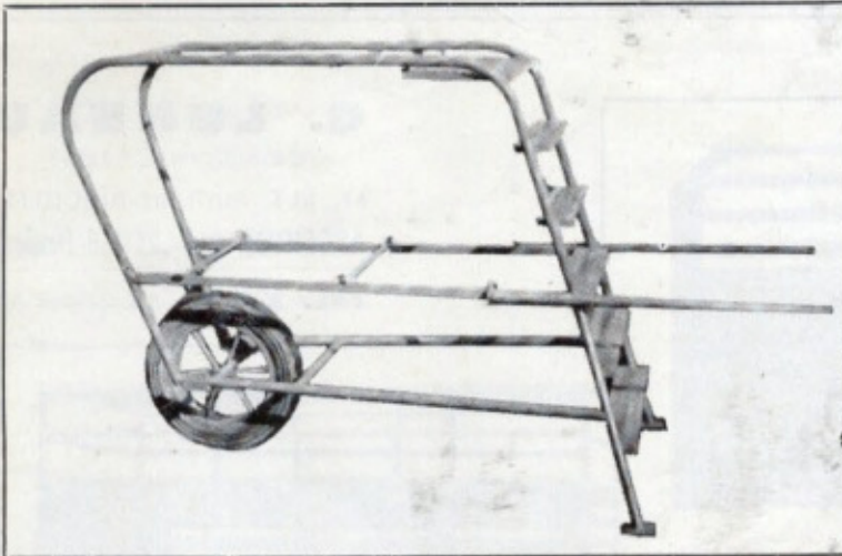
Brouette escabeau pour taillage et ramassage des fruits N° 1, 3 marches Hauteur 0 m 60 N° 2, 6 marches Hauteur 1 m 20 Peut se faire plus haute sur demande
