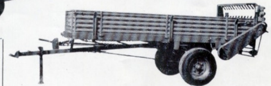
REMORQUES EN POSITION ÉPANDEUR TYPE G. L. 30 (C. U. 3 TONNES)
