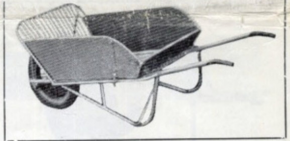
Brouette ordinaire foncée avec côtés N° 1, petite - plateau 0,50 x 0,50 roue de 350 ou 400 N° 2, moyenne - plateau 0,60 x 0,50 roue de 350 ou 400 N° 3, grosse - plateau 0,70 x 0,52 roue de 400 ou 500
