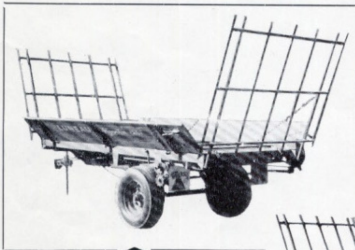
Remorque transformée en Fourragère élargie à 2 m 20
