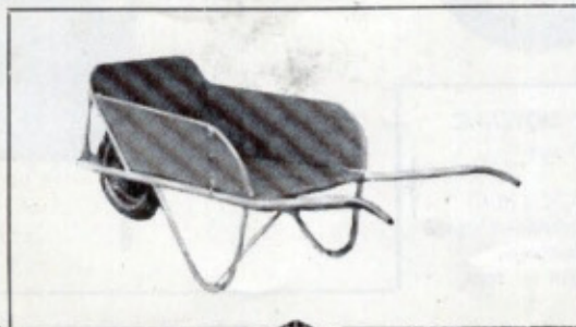
Brouette ordinaire foncée avec côtés N° 1, petite - plateau 0,50 x 0,50 roue de 350 ou 400 N° 2, moyenne - plateau 0,60 x 0,50 roue de 350 ou 400 N° 3, grosse - plateau 0,70 x 0,52 roue de 400 ou 500
